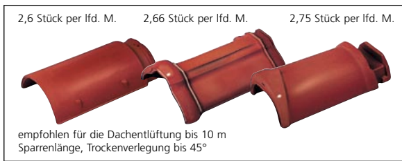
Firstziegel Nr. 15
